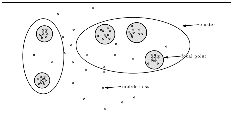
Fig. 1. Clusters
